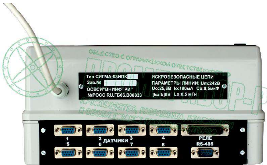
Рис.1. Внешний вид блока информационного СИГМА-03.ИПК
